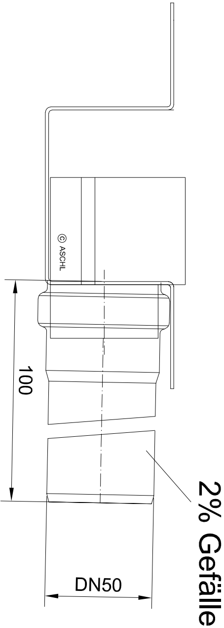
Schnitt B-B
