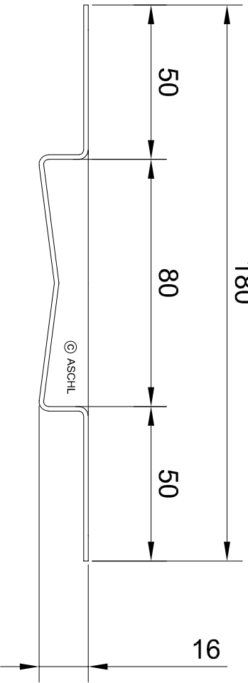
Schnitt A-A
